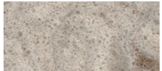
3017 Milky Way
